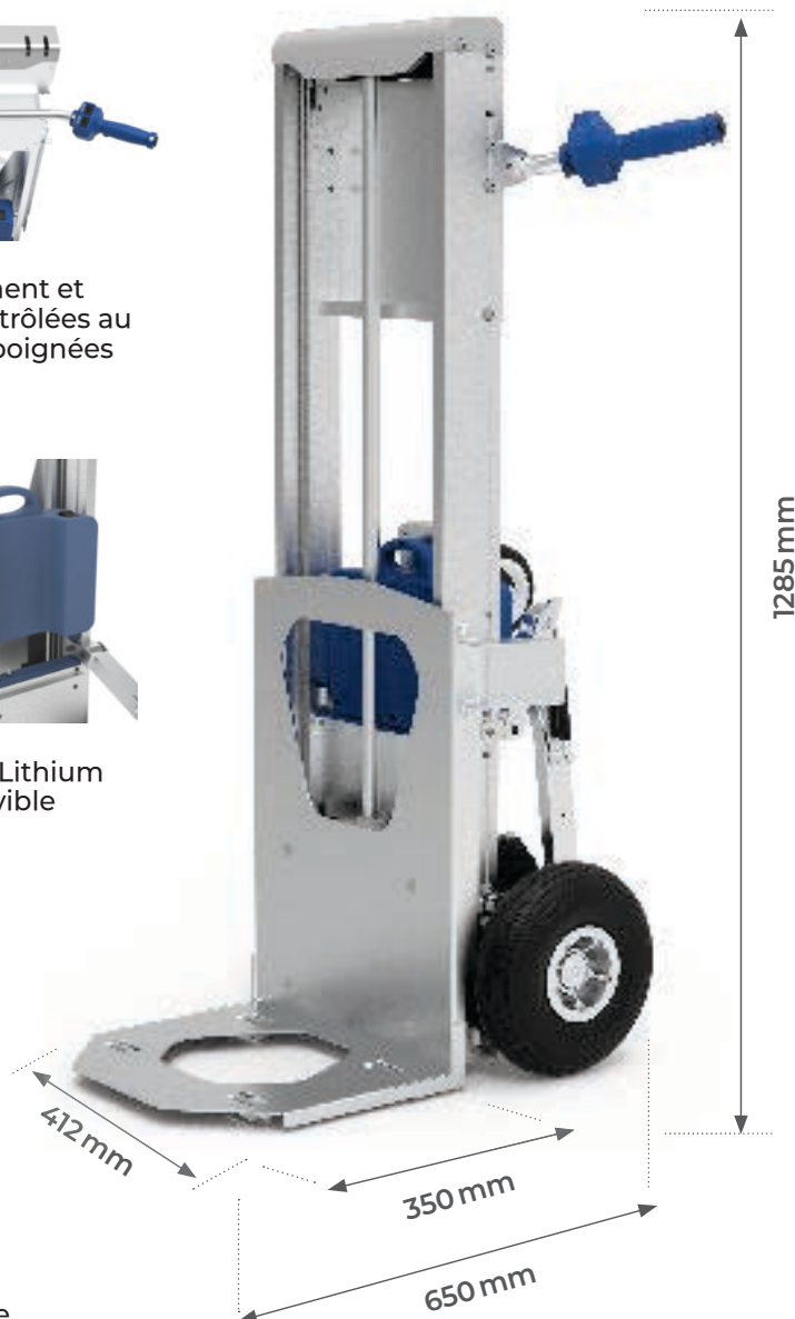
Roue auxiliaire rabattable
